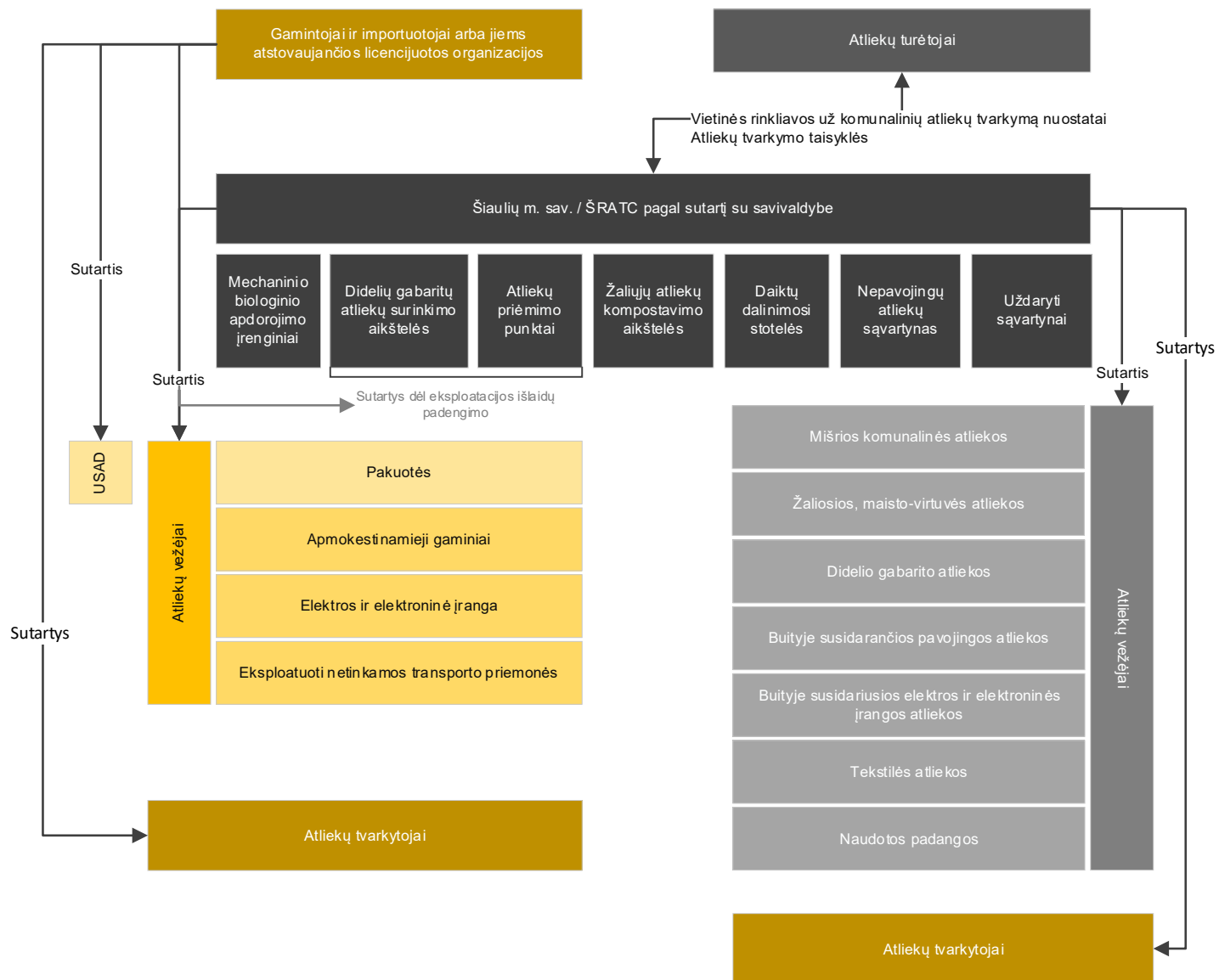
1 paveikslas. Šiaulių m. sav. komunalinių atliekų tvarkymo sistemos organizacinė schema
