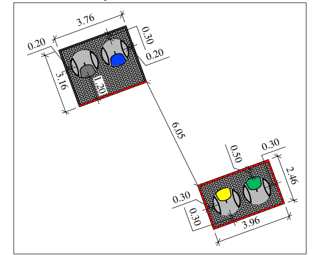
Aikštelės detalizacija
