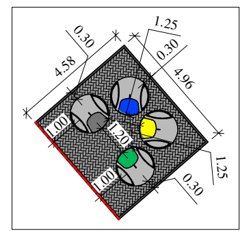
Aikštelės detalizacija
