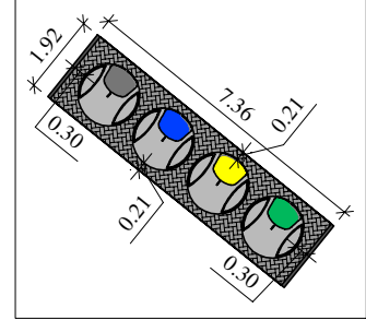
Aikštelės detalizacija
