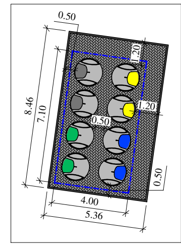
Aikštelės detalizacija
