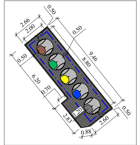
Aikštelės detalizacija
