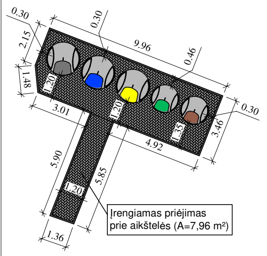
Aikštelės detalizacija
