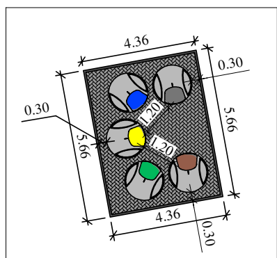
Aikštelės detalizacija
