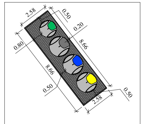
Aikštelės detalizacija
