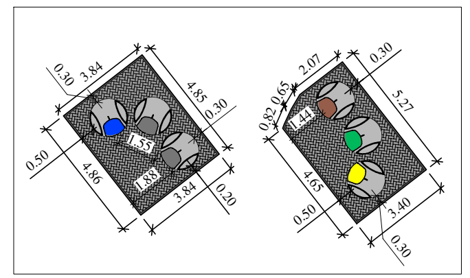
Aikštelės detalizacija
