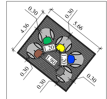
Aikštelės detalizacija
