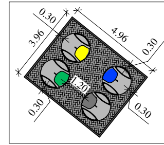
Aikštelės detalizacija
