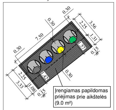
Aikštelės detalizacija
