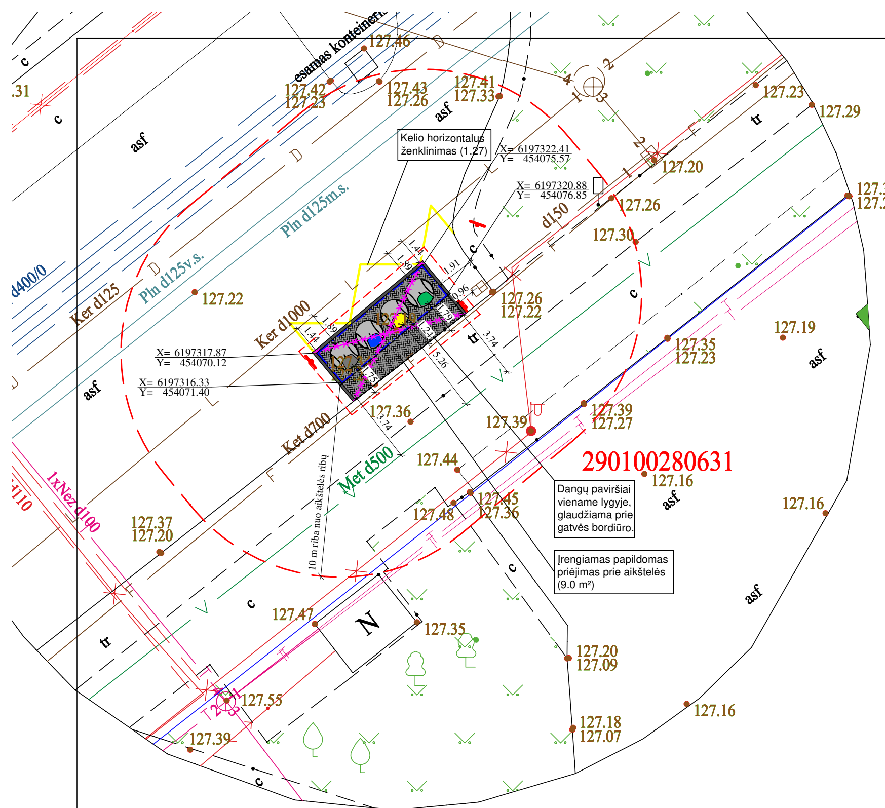
Aikštelės detalizacija
