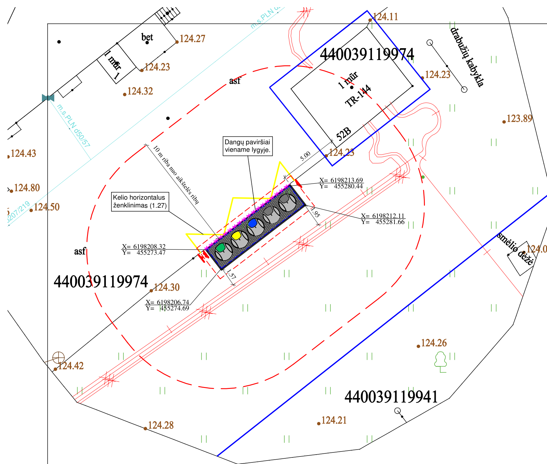
Aikštelės detalizacija
