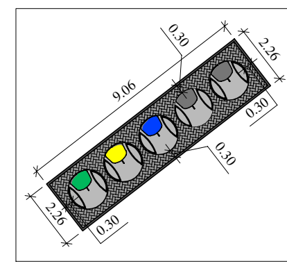
Aikštelės detalizacija
