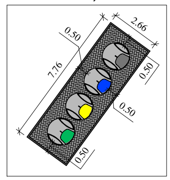
Aikštelės detalizacija
