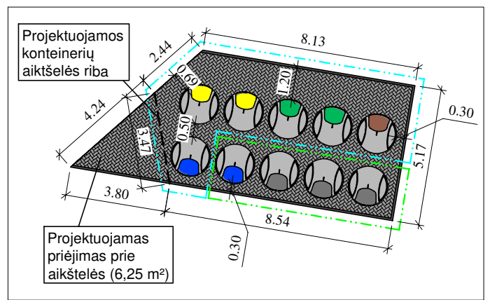
Aikštelės detalizacija
