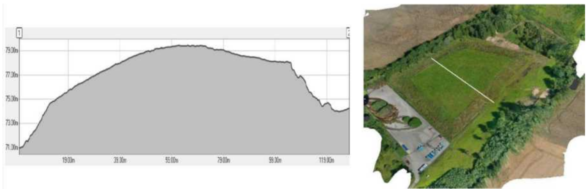
17 pav. uždaryto Aleknaičių sąvartyno, taikant fotogrametrinius metodus ir bepiločius orlaivius, skersinis pjūvis
